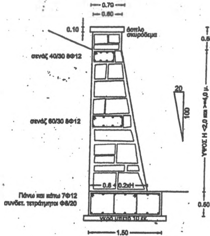
ΤΟΙΧΟΣ ΤΥΠΟΥ Β από 2,0 μέχρι 4,0 μ. κλ. 1:50
