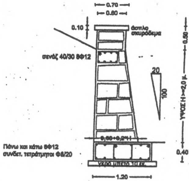
ΤΟΙΧΟΣ ΤΥΠΟΥ Α μέχρι 2,0 μ. κλ. 1:50
