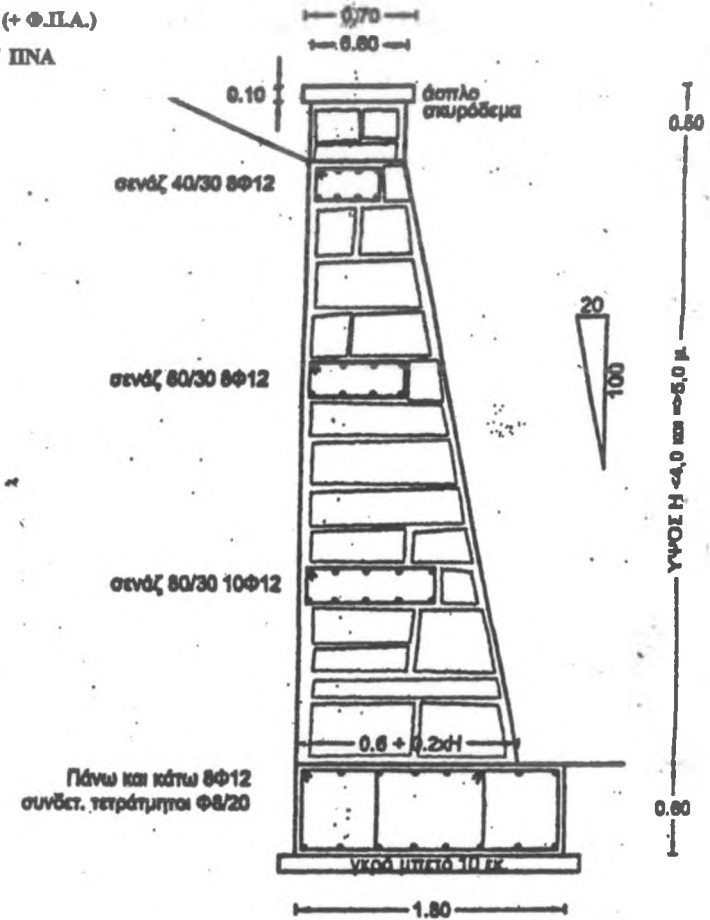
ΤΟΙΧΟΣ ΤΥΠΟΥ Γ από 4,0 μέχρι 5,0 μ. κλ. 1:50
